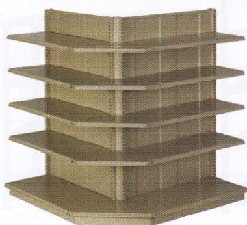
SP - 310 F 1384W x 460D x 1489H mm.
