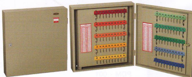
KB - 8200 530W x 110D x 550H mm.
